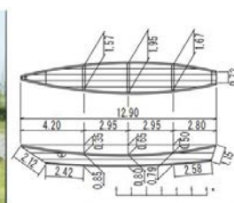
高瀬舟の基準図（明治15年までの標準型）
